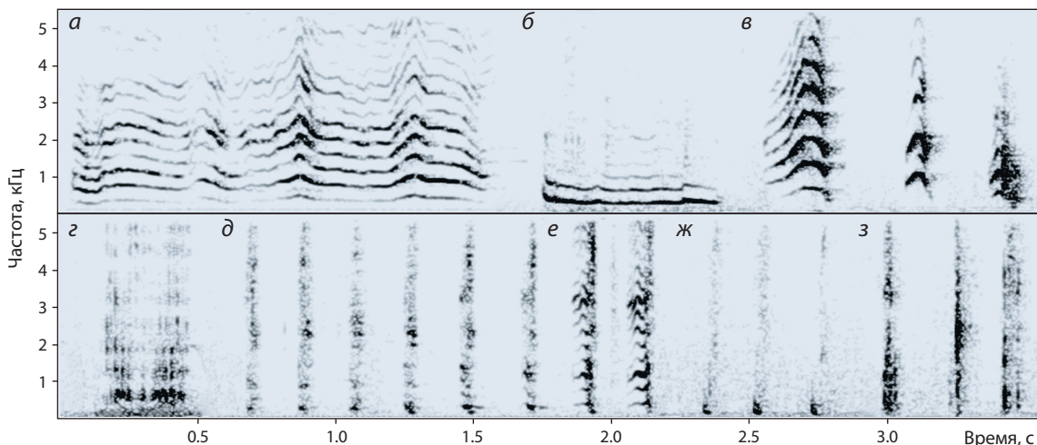
Рис. 1. Спектрограммы восьми типов звуков лисиц: скуление (а), мычание (б), лай (в), рычание (г), шумное дыхание (д), кудаханье (е), фыркание (ж), кашель (з).
