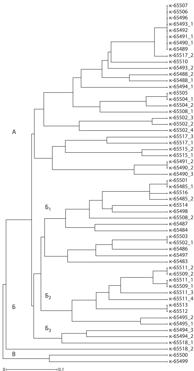
Сходство электрофоретических спектров глина 58 биотипов СГП. Дендрограмма построена с использованием UPGMA-метода.
