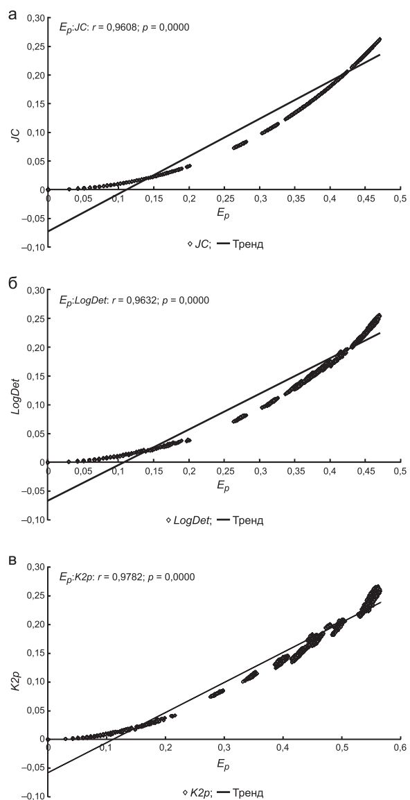
Рис. 1. Зависимость расчетных генетических расстояний от их наблюдаемых аналогов.
