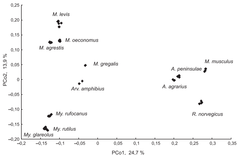
Рис. 2. Расположение нуклеотидных последовательностей на плоскости I–II главных координат.
