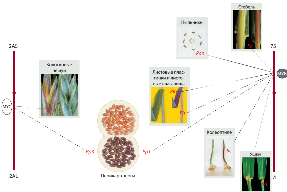
Рис. 5. Хромосомная локализация генов пшеницы, детерминирующих антоциановую окраску и кодирующих регуляторные факторы MYC- и MYB-типа.
