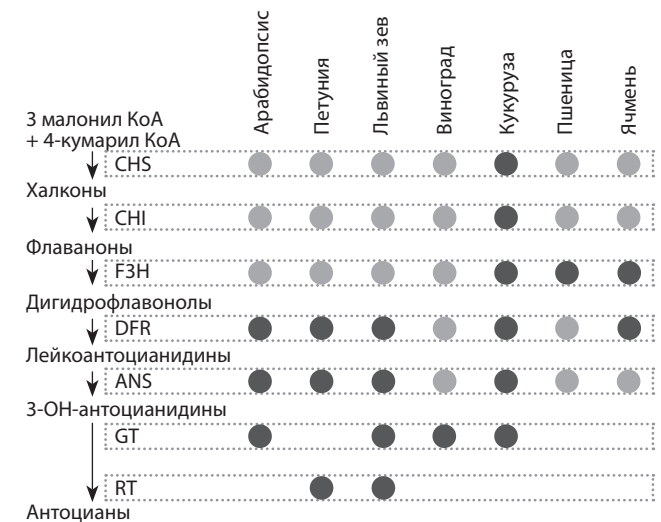
Рис. 4. Активность структурных генов биосинтеза антоцианов в окрашенных (темные круги) или неокрашенных (светлые круги) антоцианами тканях у представителей двудольных и однодольных.
