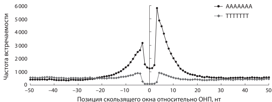
Рис. 4. Профили встречаемости поли-А трактов длины 7 нт в участках, содержащих ОНП в геноме человека.
