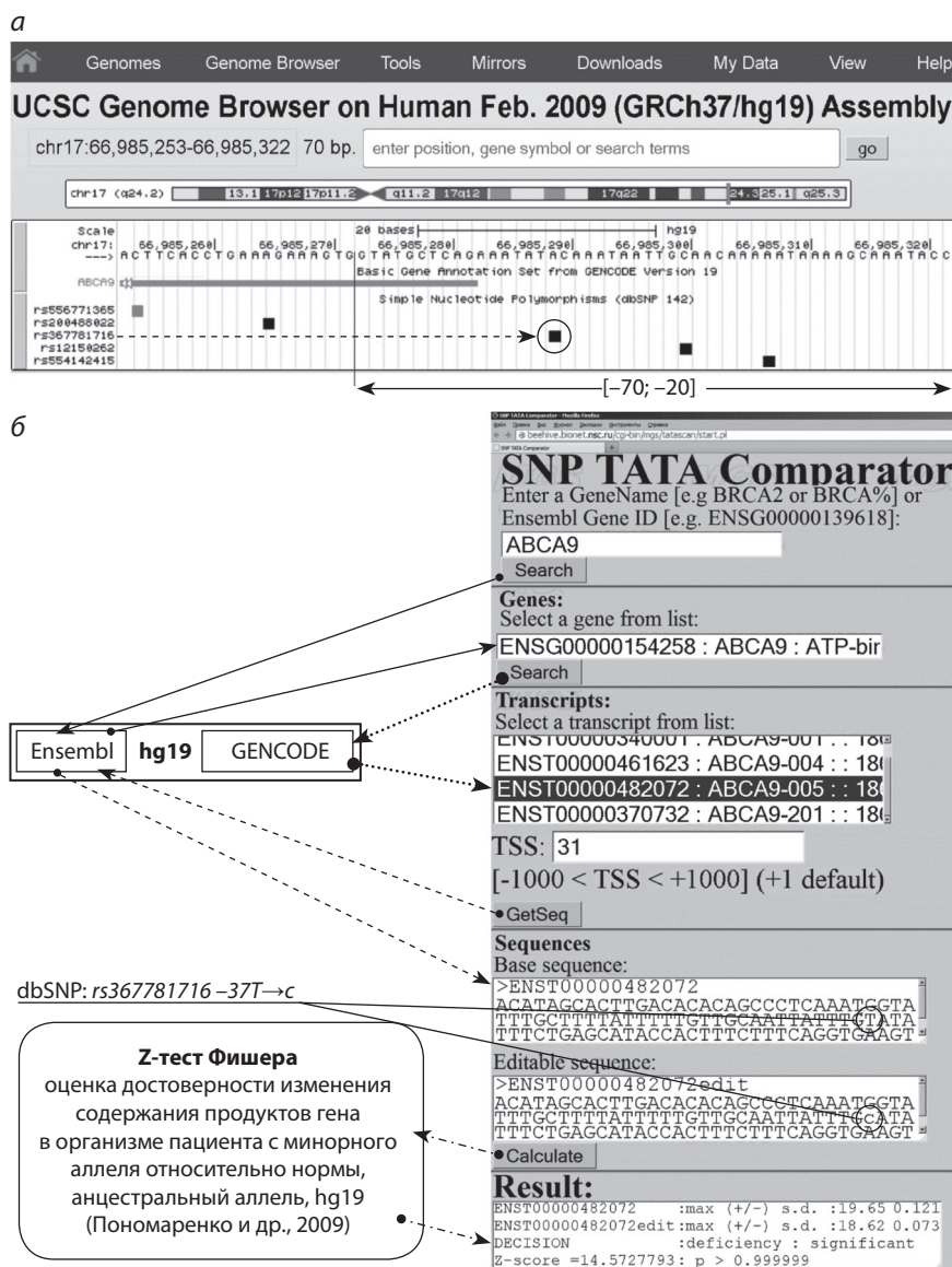
Рис. 1. Локализация (а) неаннотированного SNP rs367781716, замена -37T→C в промоторе гена ABCA9 человека и (б) его компьютерный анализ с помощью Web-сервиса SNP_TATA_Comparator (Рассказов и др., 2013).
