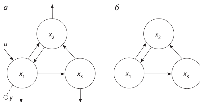
Рис. 4. Трехкамерная фармакокинетическая линейная модель (а), u – функция ввода препарата, y – измерения из первой камеры. Граф с тремя вершинами (б).
